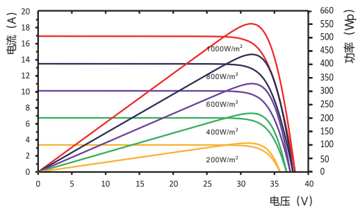
不同辐照度下, I-V曲线图
