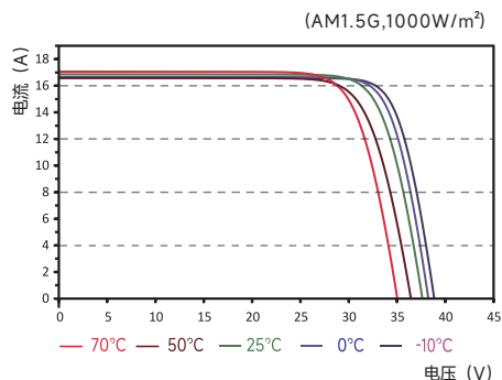
不同电池温度下, I-V曲线图
